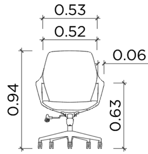
elevação frontal
