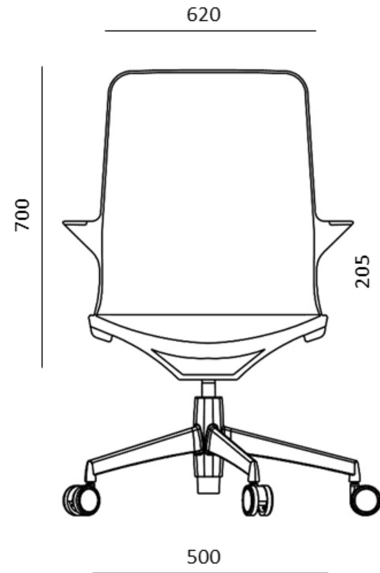
elevação frontal
