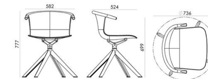
elevação frontal elevação lateral vista superior
