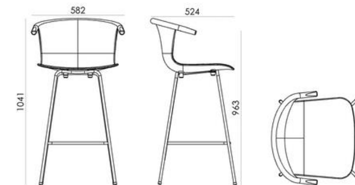
elevação frontal elevação lateral vista superior
