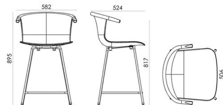
elevação frontal elevação lateral vista superior
