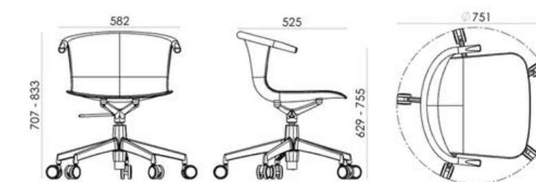
elevação frontal elevação lateral vista superior
