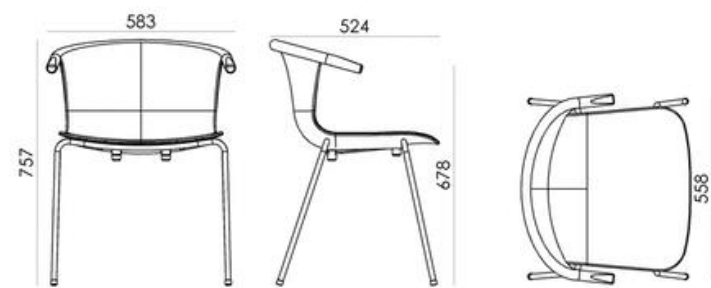
elevação frontal elevação lateral vista superior
