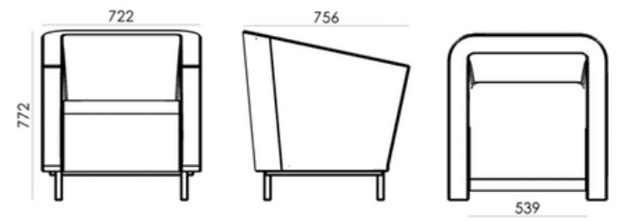
elevação frontal elevação lateral vista superior
