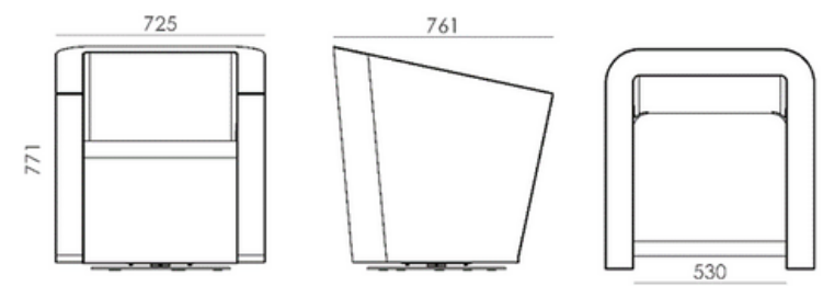
elevação frontal elevação lateral vista superior
