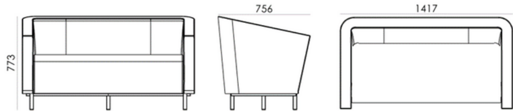
elevação frontal elevação lateral vista superior
