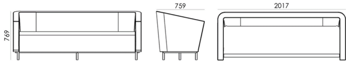
elevação frontal elevação lateral vista superior
