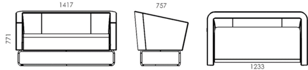
elevação frontal elevação lateral vista superior
