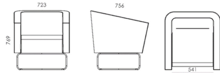
elevação frontal elevação lateral vista superior
